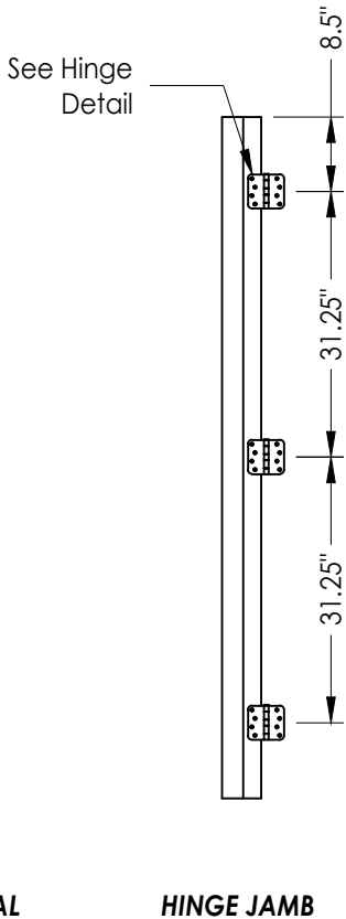
HINGE JAMB
